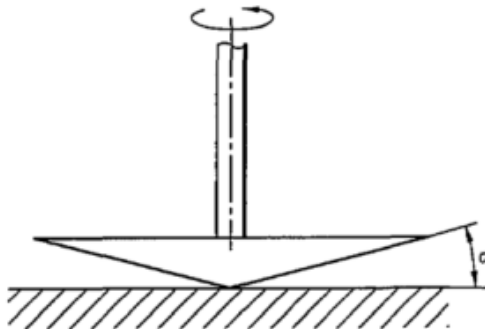
图 B.1 锥板系统
